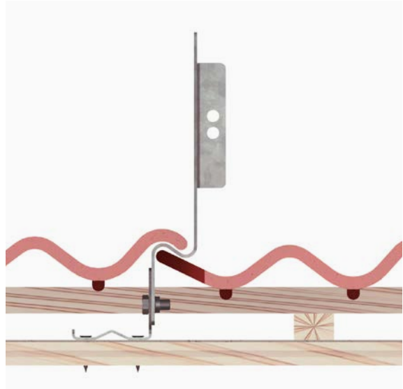
Hållare för svenskt lertegel sedd i tvärsektion.
