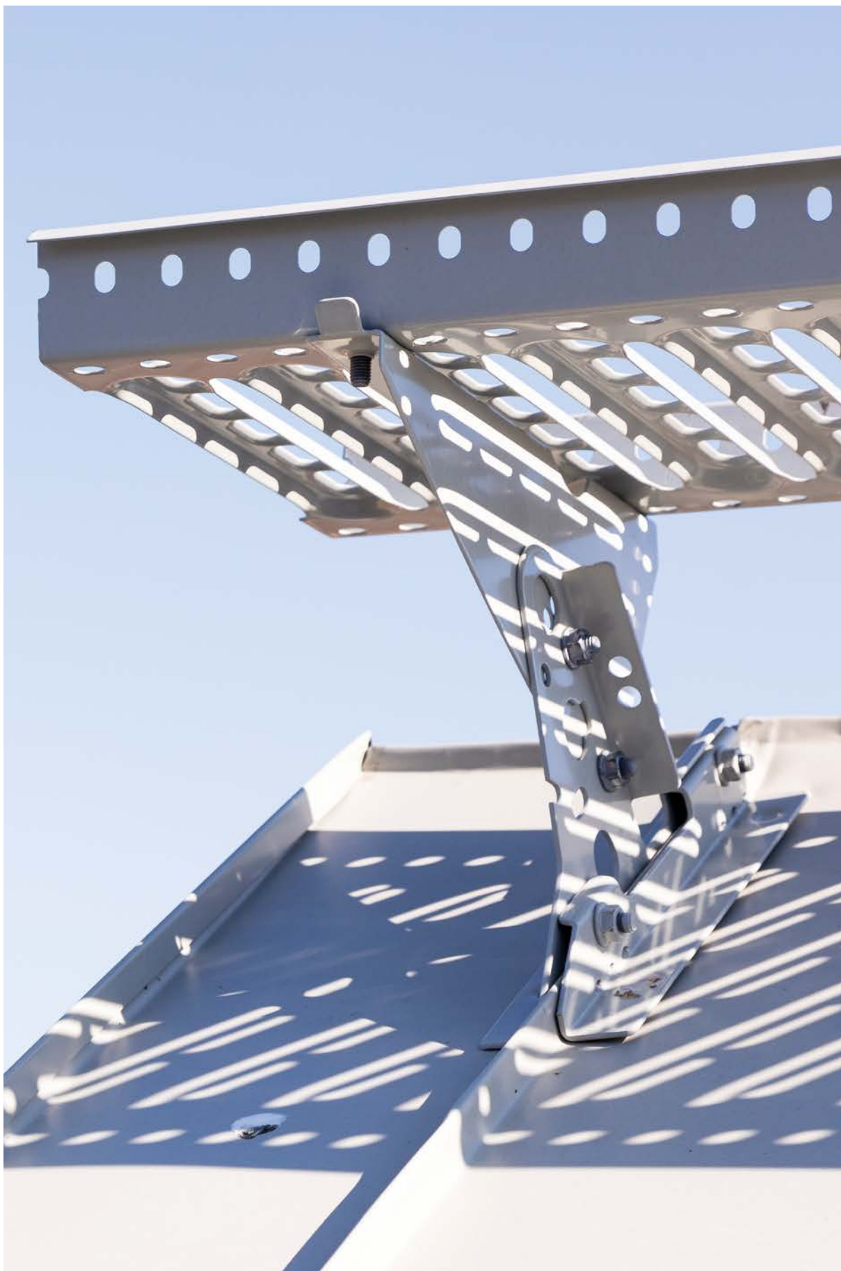
Takbrygga med falsfäste på bandtäckt tak.
