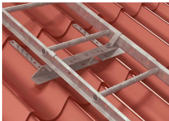
Infästningsprofil för profilerade plåttak.
