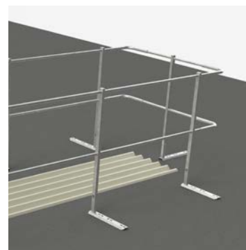
Skyddsräcke med två rör vid ljusinsläpp.
