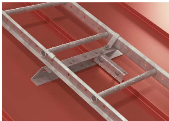
Fäste för bandtäckning.
