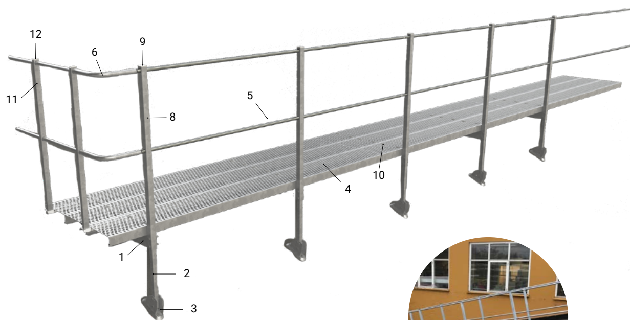
Utrymningsbrygga
