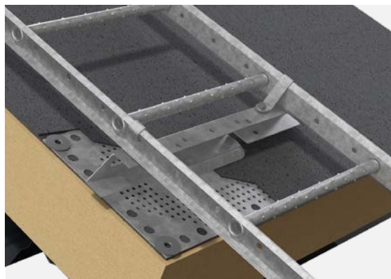
Tätplåt för tätskikt.
