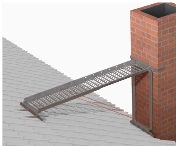
Fällbar skorstensplattform.
