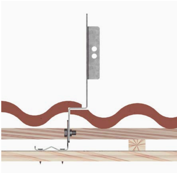
Hållare för betongpannor och falsade lertegel sedd i tvärsektion.
