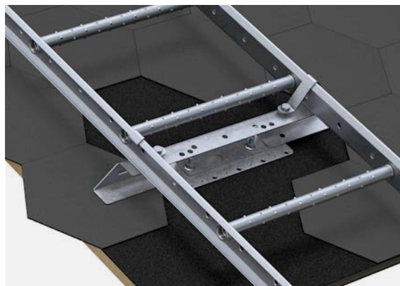
Fästplatta på shingeltak.
