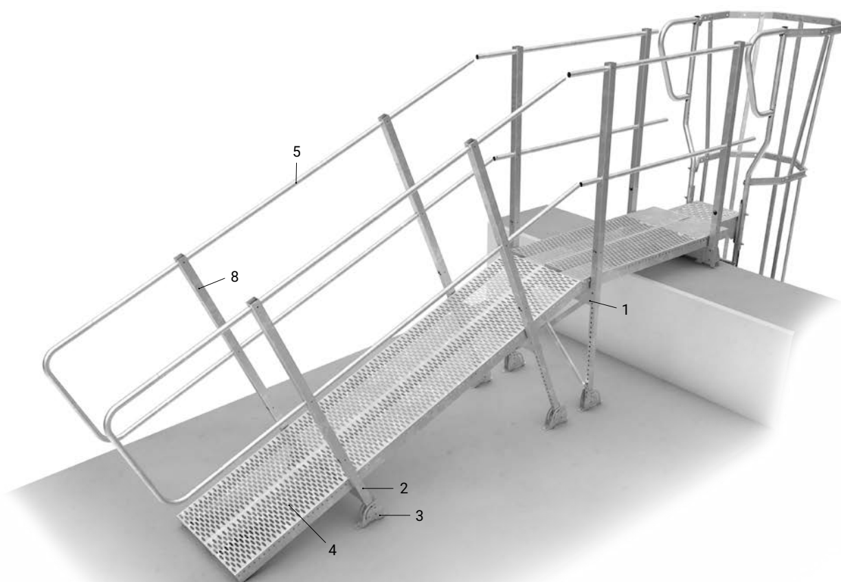
Tillträdesbrygga
