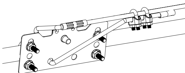
Weline ONE på mønerekkverk
