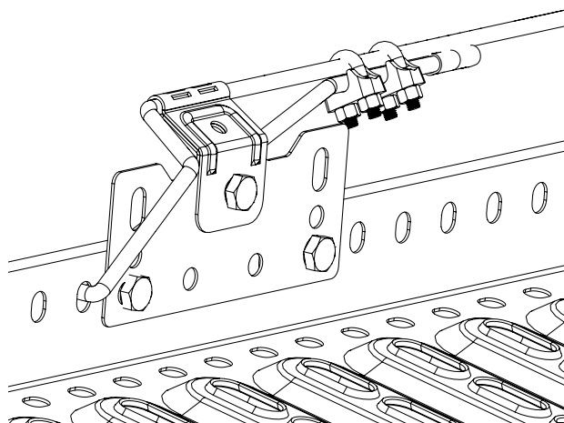
Weline ONE på takbro
